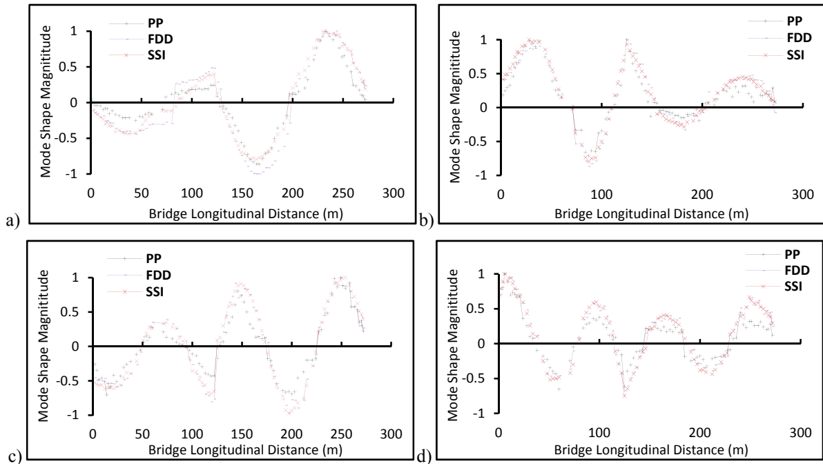
Figure 5. Mode shape comparison between PP, FDD and SSI: AVT a) 3L, b) 4L, c) 5L, d) 6L, e) 7L, and f) 8L; FVT g) 2V, h) 3V, i) 7V, j) 3L, k) 5L, and l) 7L
